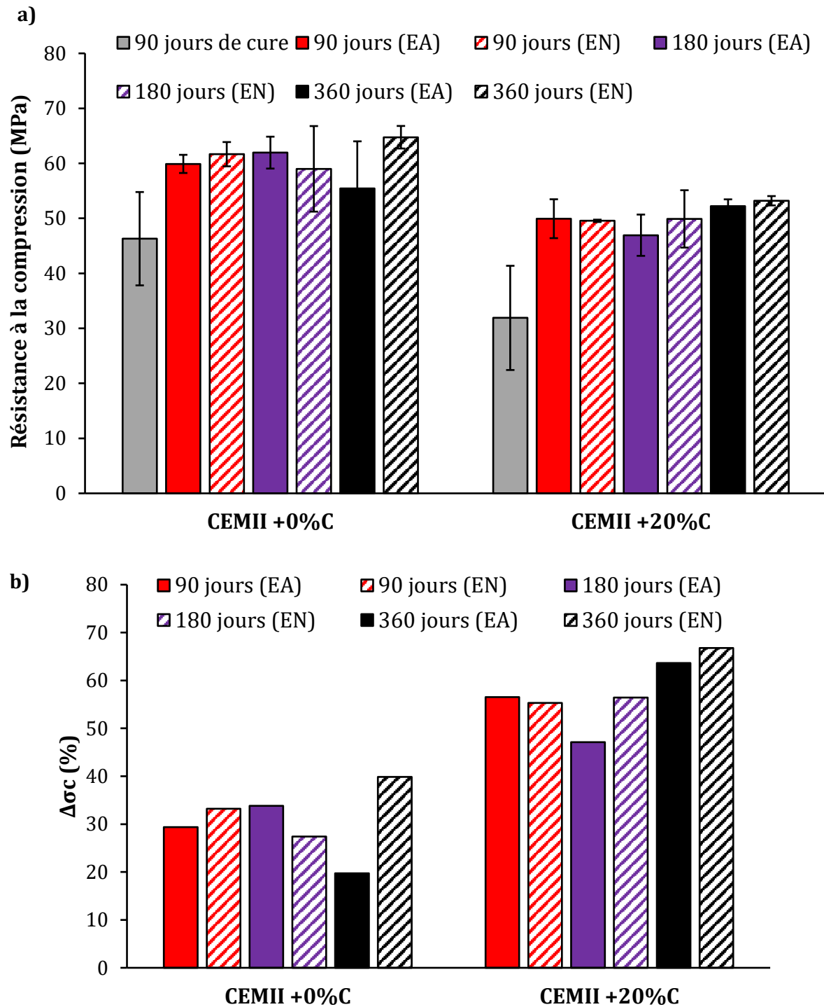
Figure 85. Résistance à la compression des bétons après 90 jours de durcissement et après 90, 180 et 360 jours d'immersion dans l'EA et l'EN (a) ; Différence relative entre les résistances à la compression respectives des bétons immergés et des bétons références (b)
