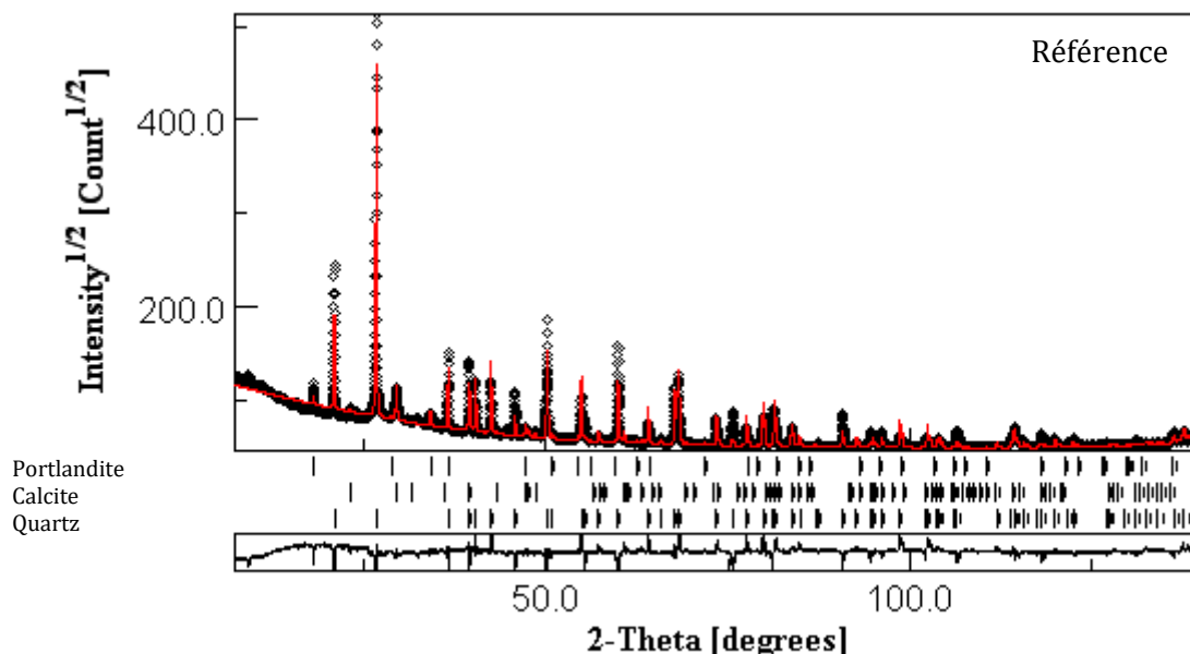
Figure 73. Spectre DRX de poudre (sur 2mm de profondeur) de mortier référence (avant immersion)
