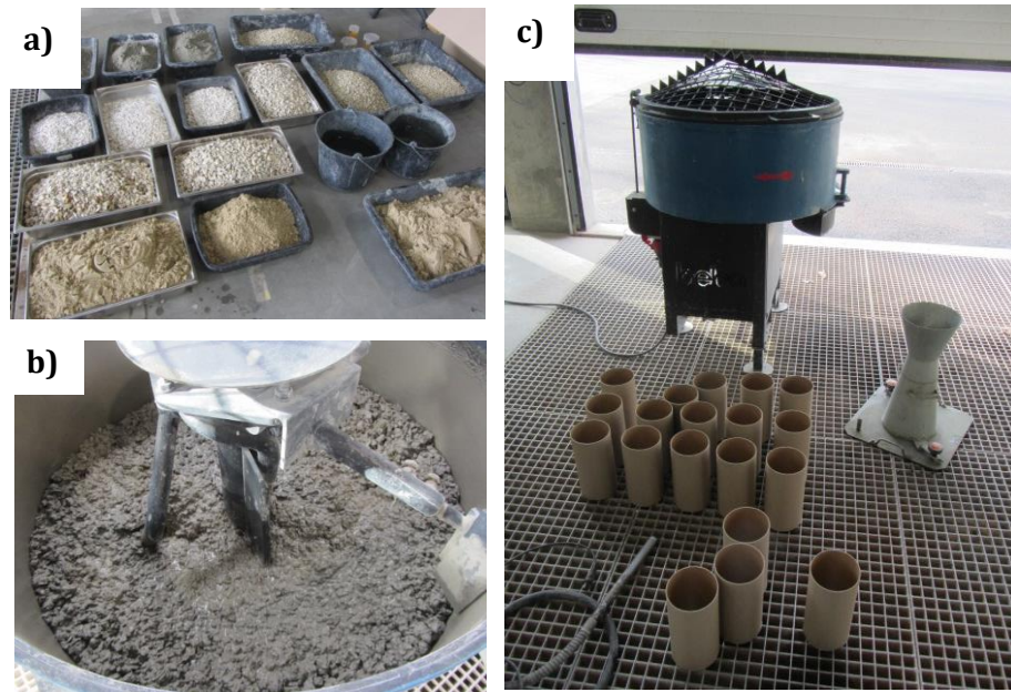
Figure 18. Préparation des constituants du béton (a) ; Malaxage du béton (b) ; Préparation du coulage (c)
