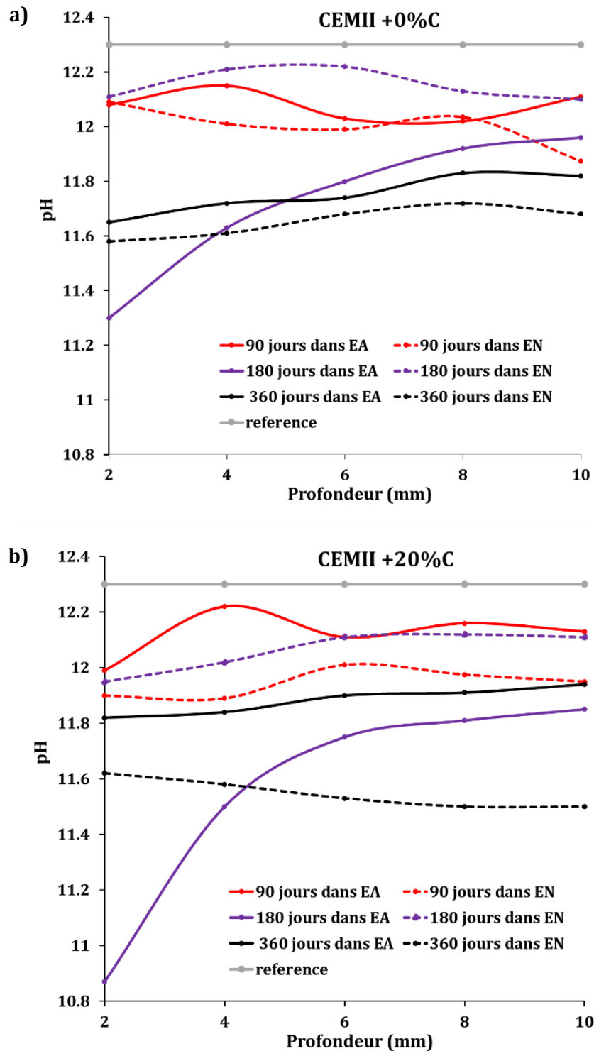
Figure 88. Variation du pH du béton CEMII +0%C (a) et CEMII +20%C (b) obtenu à partir du lixiviat de la matrice cimentaire à différentes profondeurs dans l'eau de mer naturelle (EN) et l'eau de mer artificielle (EA) après 90, 180 et 360 jours d'immersion
