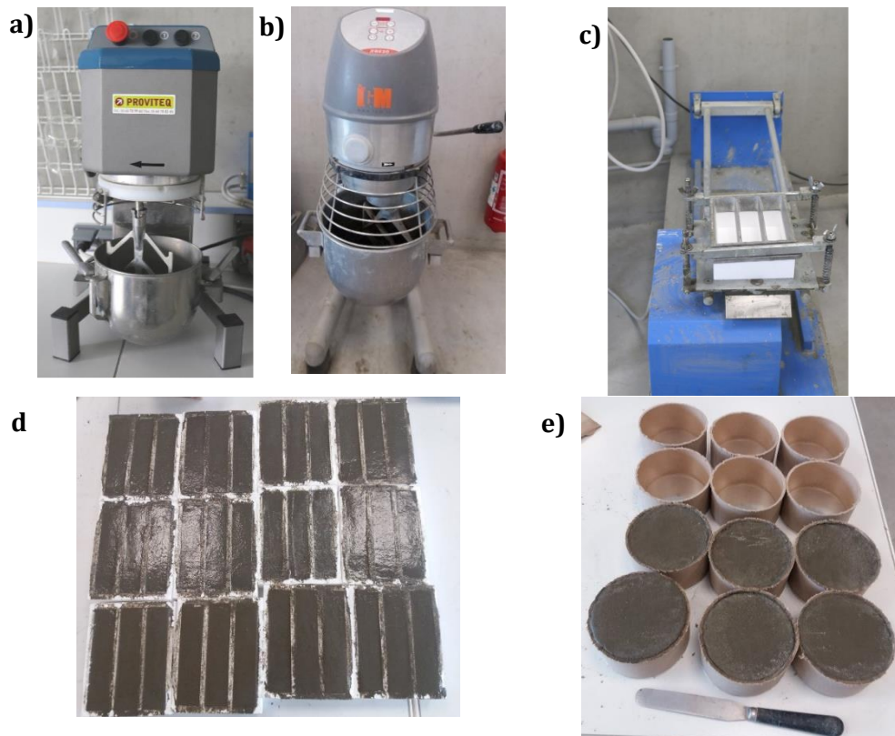
Figure 16. Malaxeurs (a) 10L et (b) 30L pour l'élaboration d'éprouvettes de mortier ; (c) table à choc et éprouvettes de mortiers (d) parallélépipédiques 40 mm × 40 mm × 160 mm et cylindriques Ø=110 mm et h=50mm
