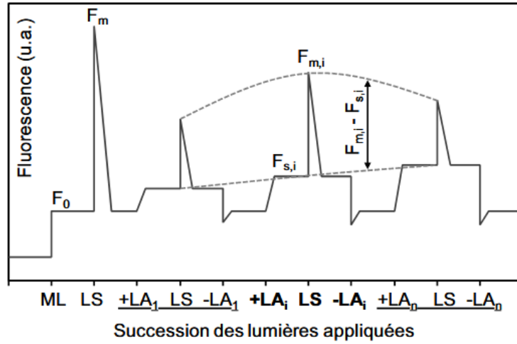
Figure 29. Schéma d'irradiation appliqué en mesure PAM (avec F_0 : rendement de fluorescence minimale après acclimatation à l'obscurité ; F_m : rendement de fluorescence maximale, d'un échantillon acclimaté à l'obscurité atteint durant un flash de lumière saturant ; F_{m,i} : rendement maximal de fluorescence d'un échantillon acclimaté à une certaine intensité lumineuse atteint durant un flash saturant ; F_{s,i} : fluorescence de base stable ; ML : Lumière de mesure de faible intensité ; LAi : Lumière actinique)
