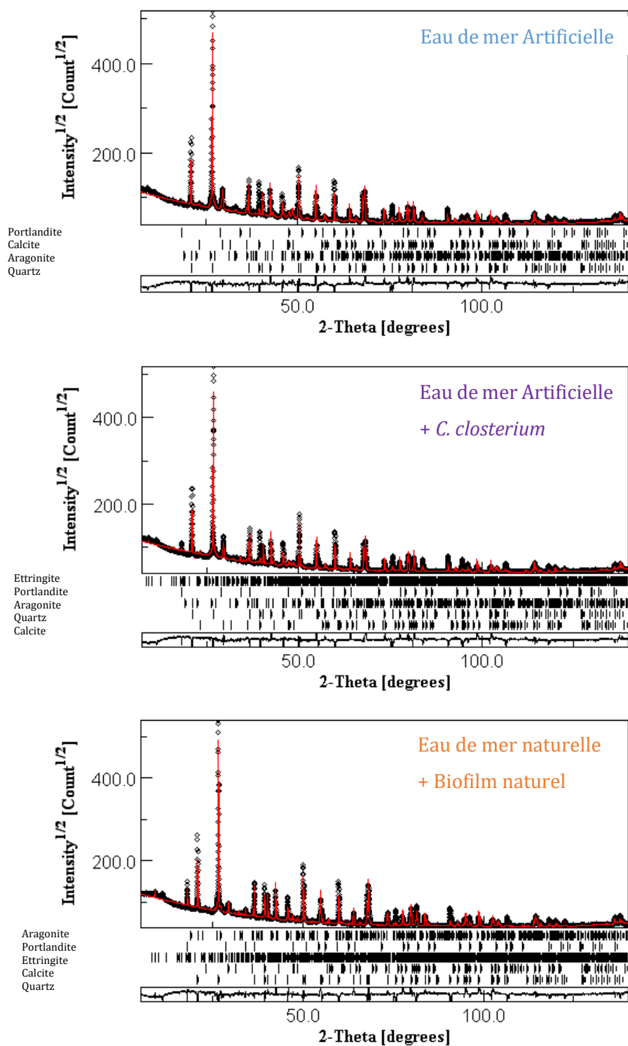
Figure 75. Spectres DRX de poudre de mortier immergé après 360 jours d'immersion dans les trois conditions étudiées (EA, EAC et EN)
