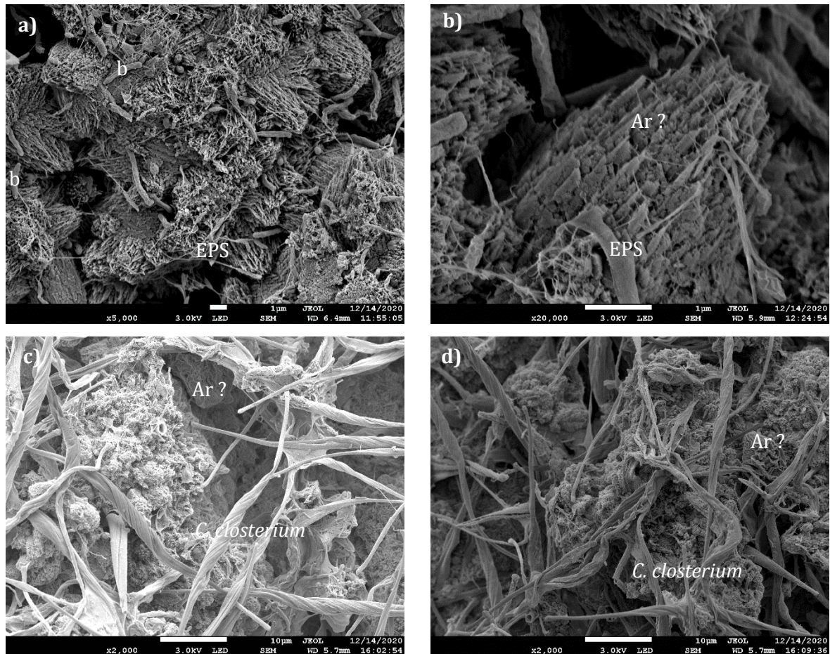
Figure 68. Observations MEB du mortier immergé en Eau de mer Artificielle avec C. closterium après 90 (a et b) et 360 jours d'immersion (c et d)
