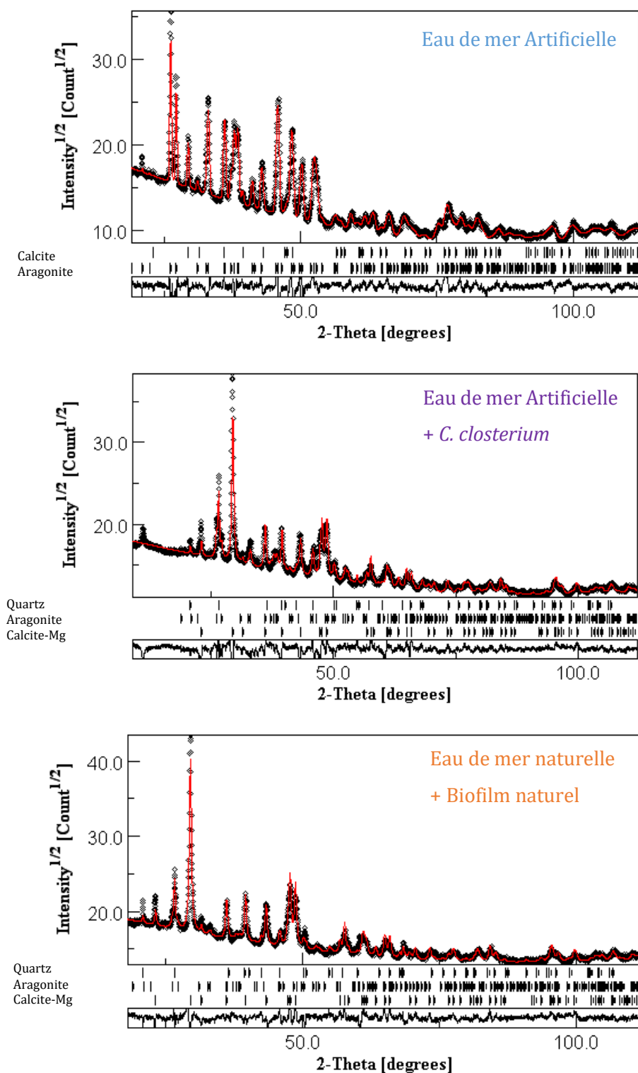
Figure 71. Spectres DRX de la surface des mortiers immergés 90 jours dans les trois conditions étudiées (EA, EAC et EN)
