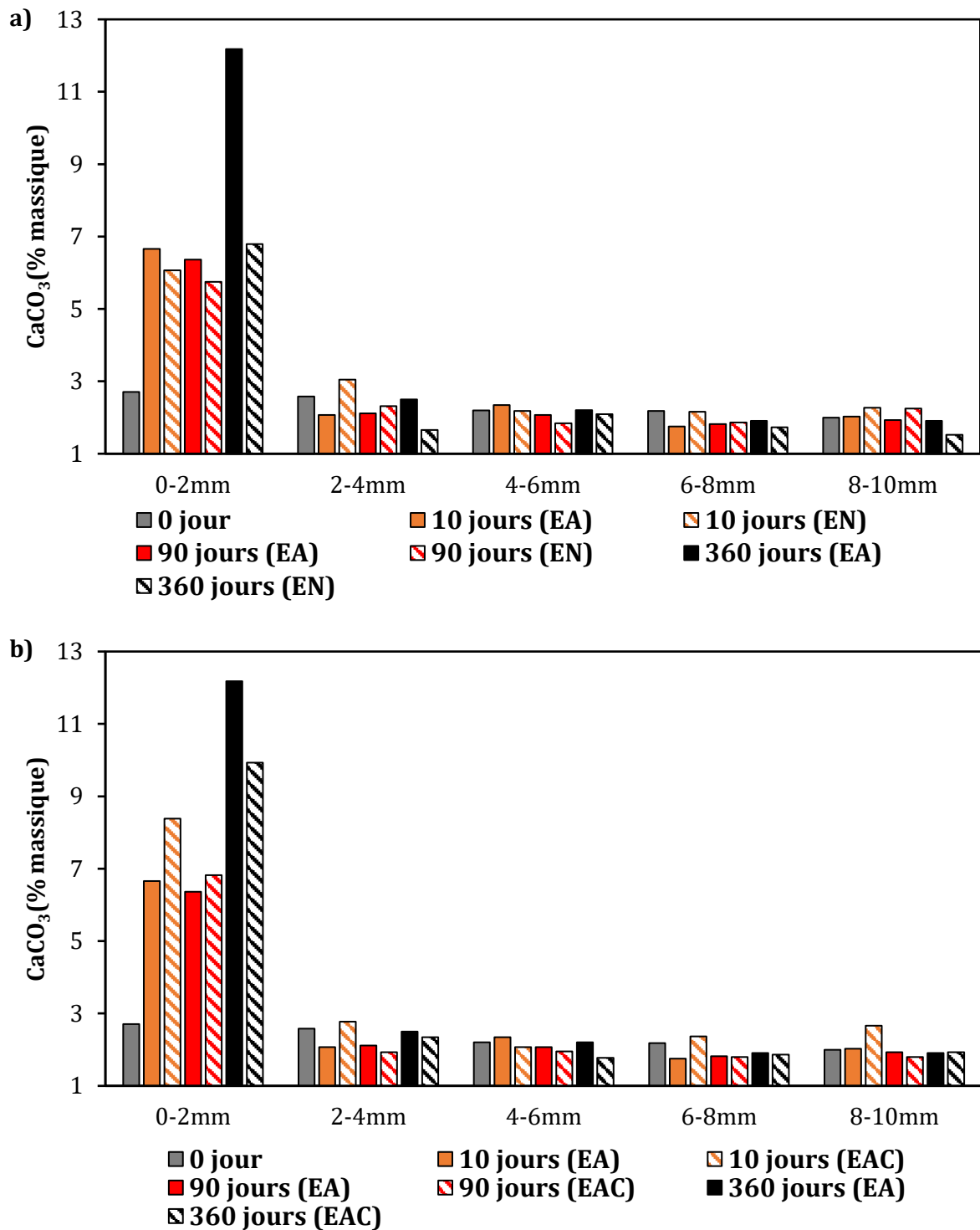
Figure 64. Evolution du Carbonate de Calcium (% massique) dans les mortiers immergés en Eau de mer Naturelle + Biofilm naturel (EN) (a) et en Eau de mer Artificielle avec C. closterium (EAC) (b) comparé au mortier référence et immergé en Eau de mer Artificielle (EA) à différentes profondeurs après 10, 90 et 360 jours d'immersion
