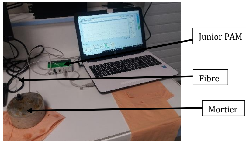
Figure 28. Mesure PAM à la surface du matériau
