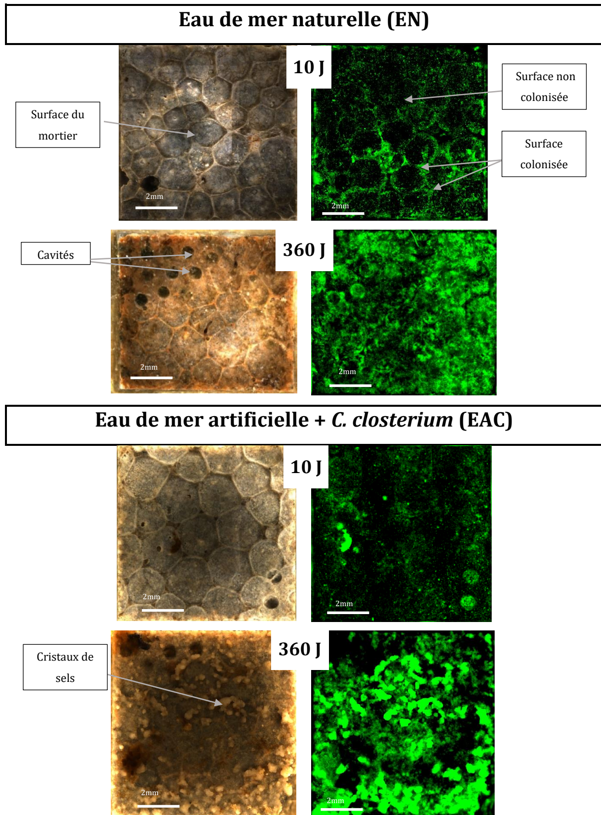
Figure 54. Observations macroscopiques (X80) de mortiers (10 mm × 10 mm × 5 mm) immergés à 10 et 360 jours (à gauche) ; Observations macroscopiques par fluorescence EGFP (à droite) en EN et EAC, la couleur verte est spécifique au pigment chlorophyllien du microphytobenthos fixé sur les échantillons, le noir représente la zone du mortier non colonisé
