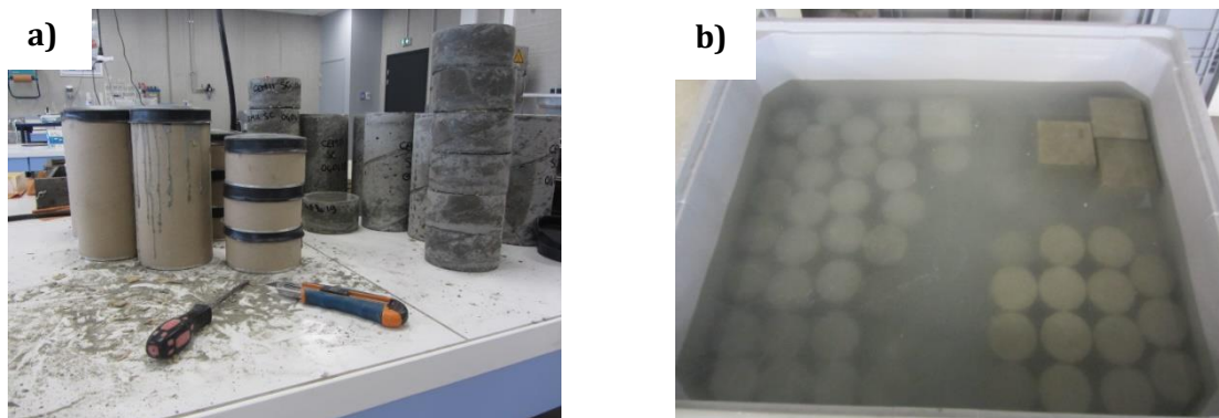
Figure 19. Démoulage des éprouvettes de bétons (a) ; Cure de 90 jours des éprouvettes dans de l'eau douce (pH =7,7) (b)
