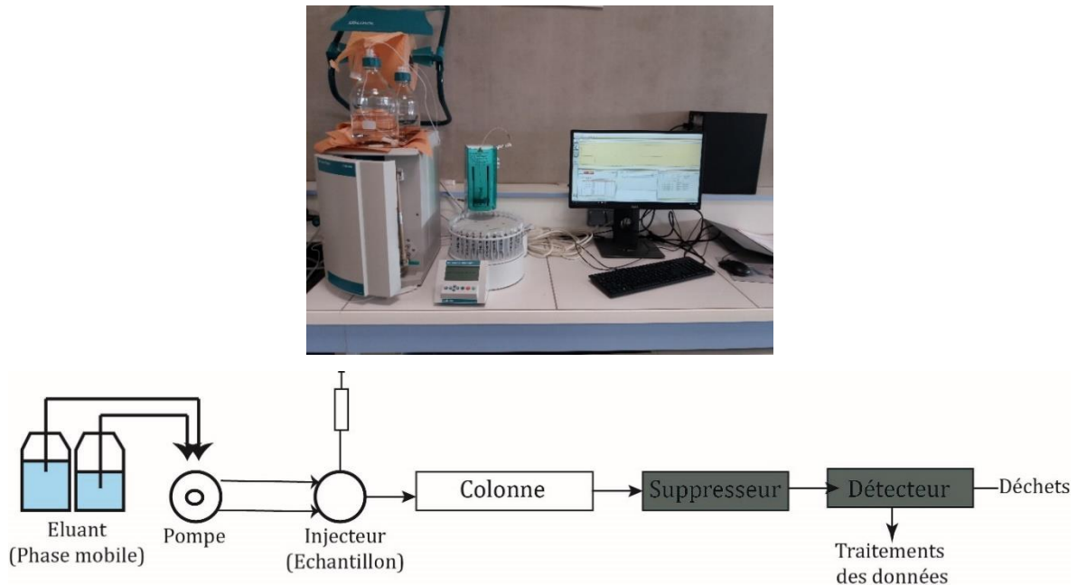
Figure 21. Chromatographe en phase ionique et son schéma de fonctionnement
