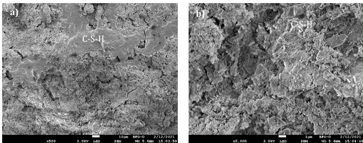
Figure 65. Observations MEB du mortier référence (avant immersion) en surface (a,b). C-S-H : gel de Calcium de Silicate Hydrate
