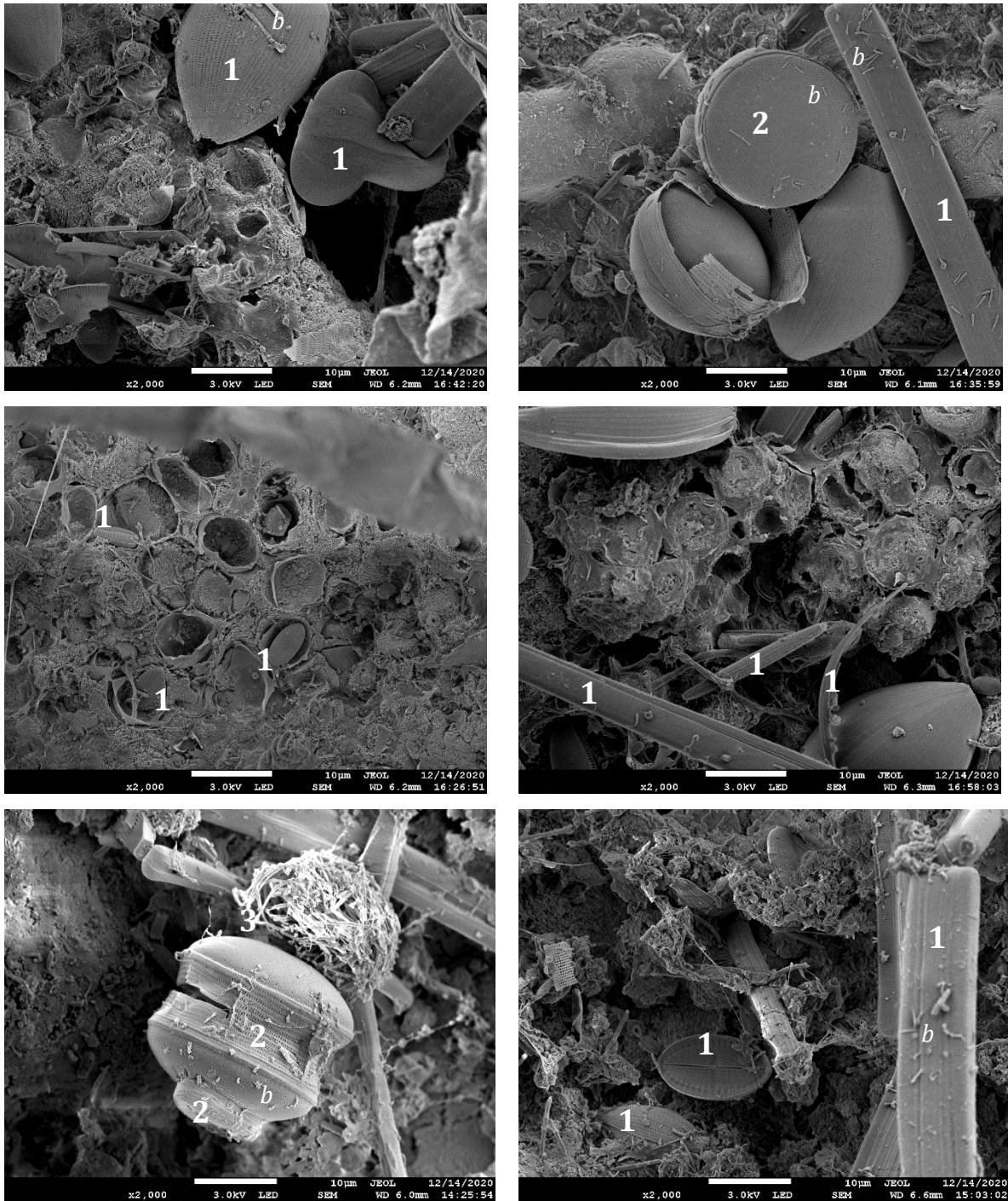
Figure 58. Exemple d'observations au Microscope Electronique à Balayage de biofilms microphytobenthiques à la surface du mortier après 360 jours d'immersion en eau de mer naturelle. Le biofilm est composé de diatomées pennales avec ou dépourvues de raphé (1), de diatomées centriques (2), de bactéries (b).
