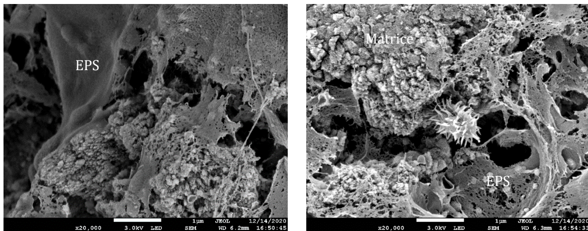
Figure 56. Exemple d'observations au microscope électronique à balayage de biofilms avec EPS (Substances Polymères Extracellulaires) sur le mortier après 360 jours d'immersion en eau de mer naturelle.
