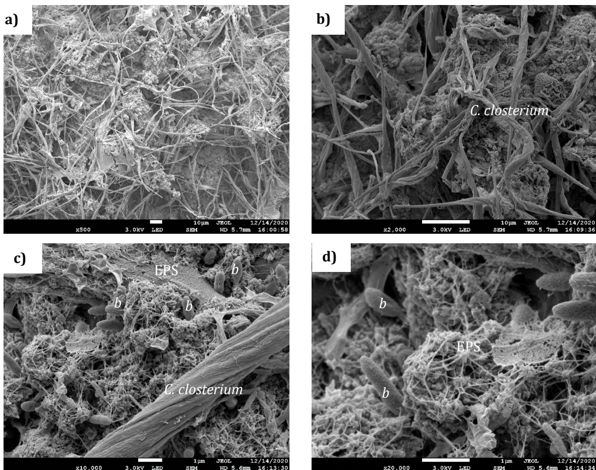
Figure 55. Exemple d'observations au microscope électronique à balayage, à différents grossissements, de biofilms de C. closterium fixés sur le mortier après 360 jours d'immersion ( a, b, c et d ) ( b : bactéries ; EPS : Substances Polymères Extracellulaires sécrétées par les micro-organismes)
