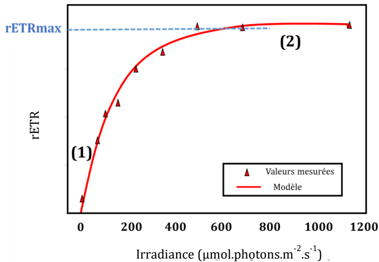
Figure 30. Courbe de réponse à la lumière rETR vs E permettant de connaître les paramètres photosynthétiques. Sur la courbe on peut observer une région limitée par la lumière, notée (1). On peut ainsi observer une région de saturation par la lumière sous forme de plateau noté (2).
