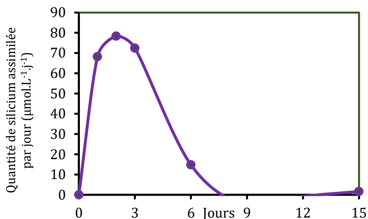
Figure 40. Si assimilée par jour par C. closterium en condition 2 (M+/Si-/Cc+).
