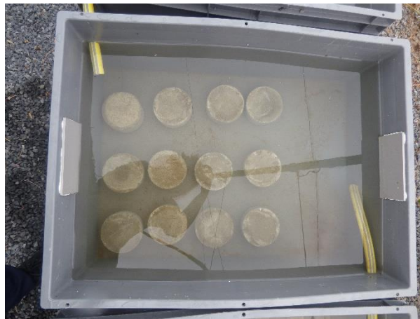
Figure 50. Dispositif expérimental des mortiers immergés dans le milieu EN
