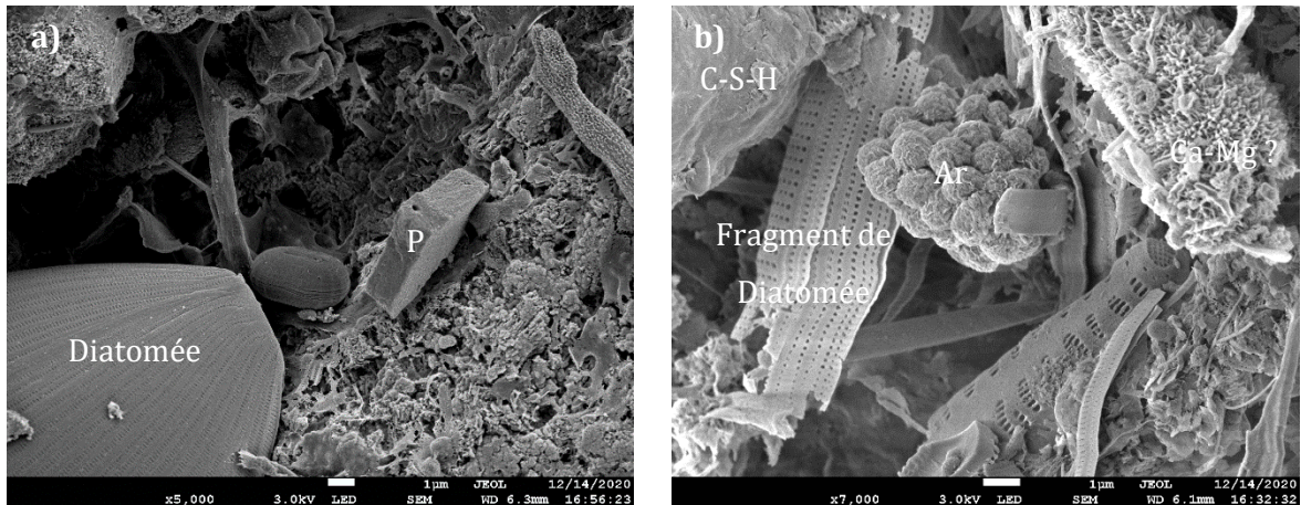
Figure 67. Observations MEB du mortier immergé en Eau de mer Naturelle après 360 jours d'immersion (a-b) (P : Portlandite, C-S-H, Ar : Aragonite, Ca-Mg : Calcite magnésienne)
