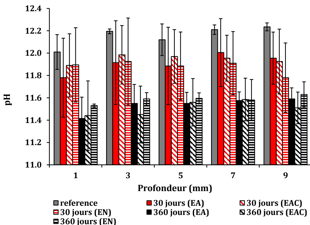
Figure 61. Evolution du pH du mortier référence et du mortier immergé après 30 et 360 jours d'immersion dans les trois milieux étudiés (EA, EAC et EN)
