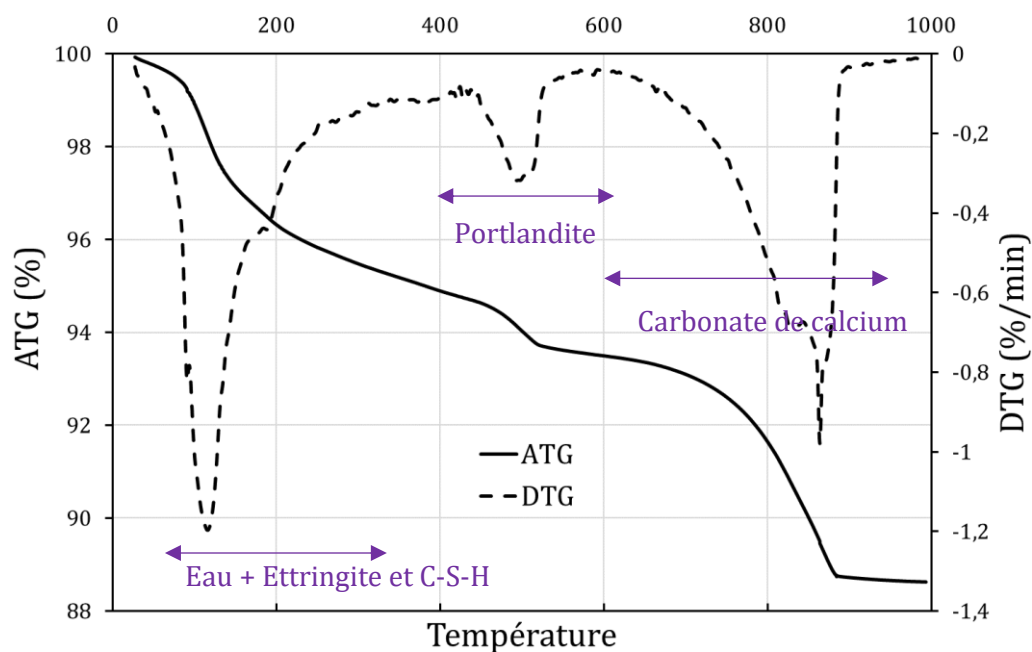
Figure 23. Courbes type ATG et DTG d'un béton coquillier après 90 jours de cure, dans les 2 premiers mm
