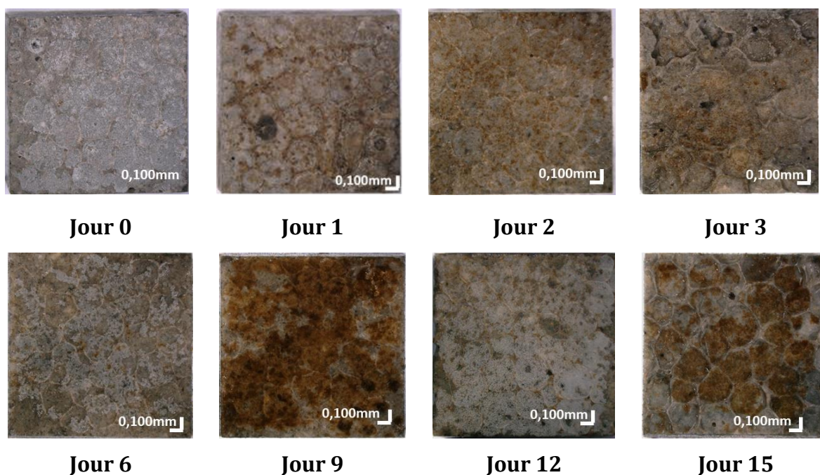
Figure 45. Exemples d'observations microscopiques (S20 x150) du mortier au jour 0, 1, 2, 3, 6, 9, 12 et jour 15 après immersion (exemple d'un des triplicats).
