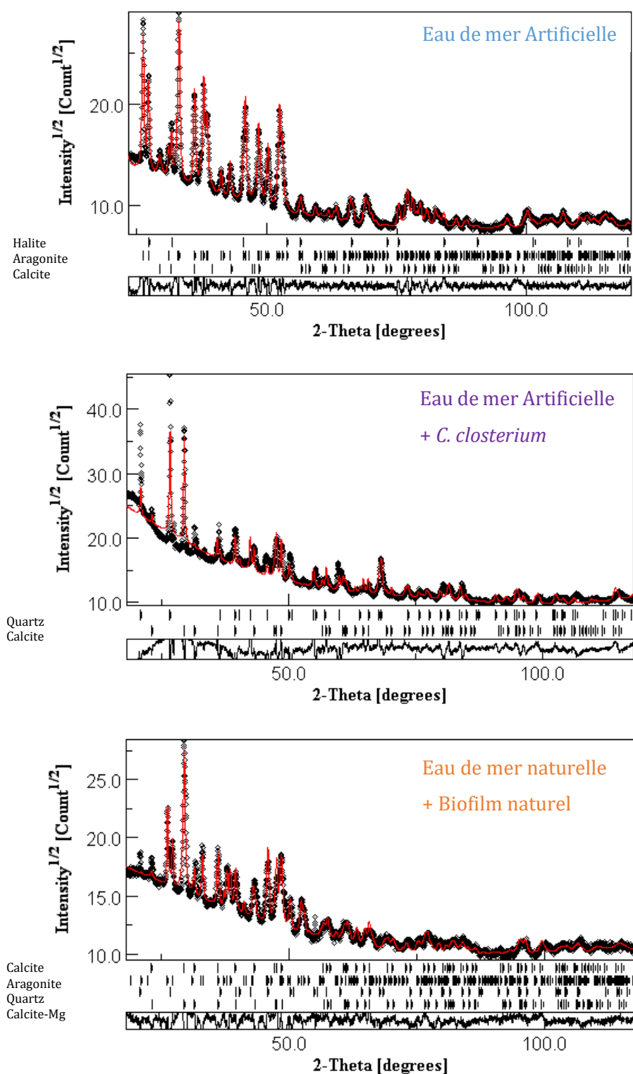
Figure 72. Spectres DRX de la surface des mortiers immergés 360 jours dans les trois conditions étudiées (EA, EAC et EN)
