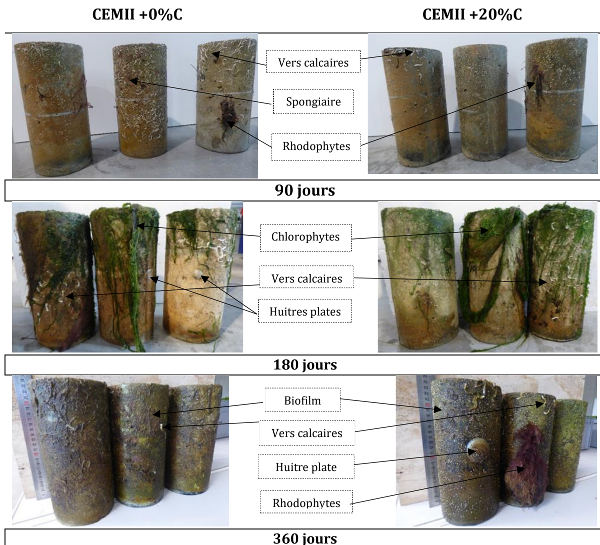
Figure 80. Photographie d'éprouvettes de béton CEMII +0%C et CEMII +20%C ( \varnothing 110 mm \times H220 mm) après 90, 180 et 360 jours d'immersion en eau de mer naturelle
