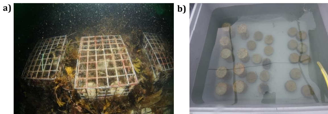
Figure 78. Immersion des échantillons de béton dans des cages pendant 3 mois dans la Rance de Dinard (a) ; immersion des échantillons en mésocosmes semi-fermés (b)
