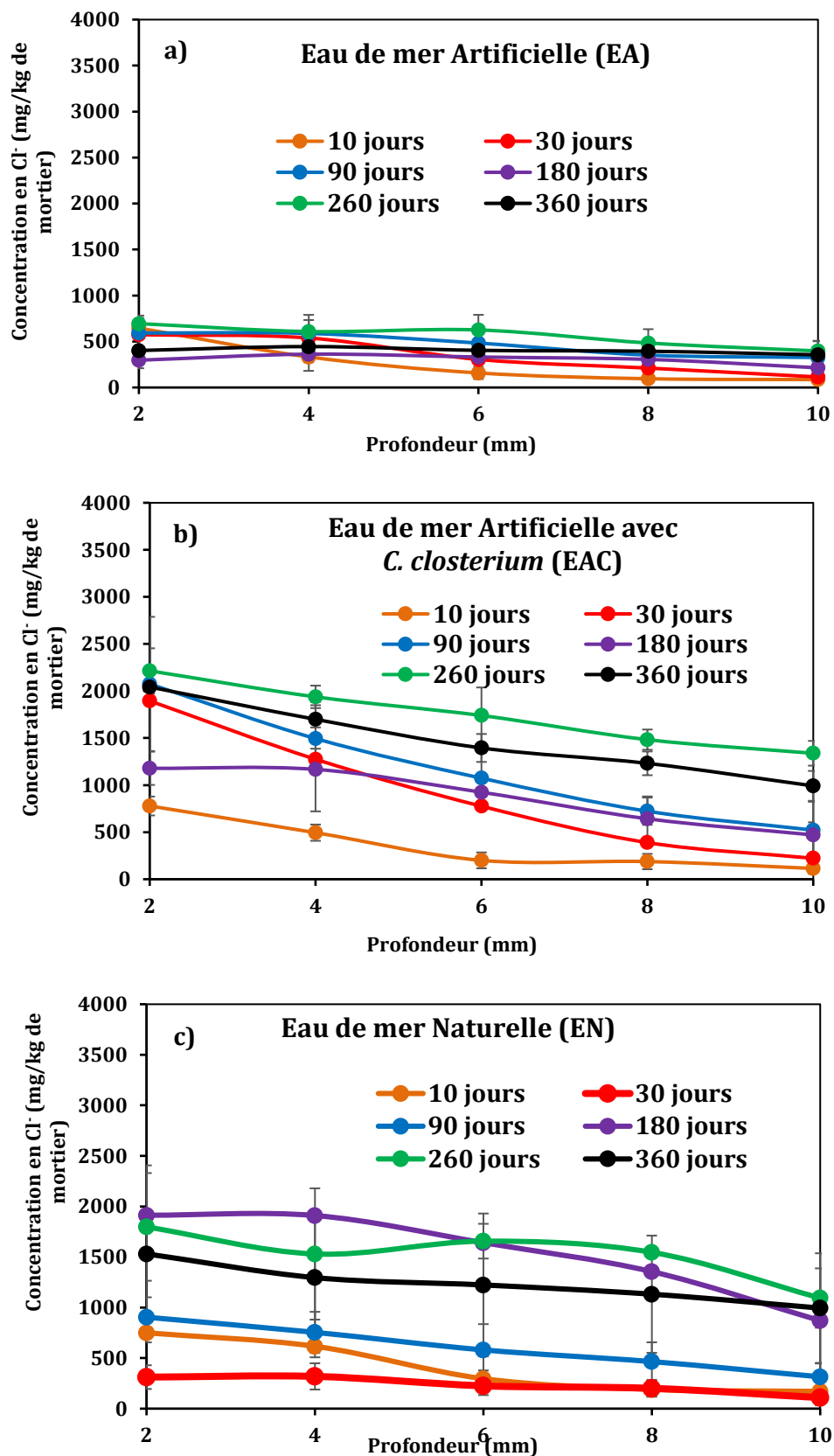
Figure 59. Diffusion des ions chlorure libres dans le mortier jusqu'à 10 mm de profondeur, au cours de l'immersion dans de (a) l'eau de mer artificielle ; (b) l'eau de mer artificielle + C. closterium ; (c) l'eau de mer naturelle
