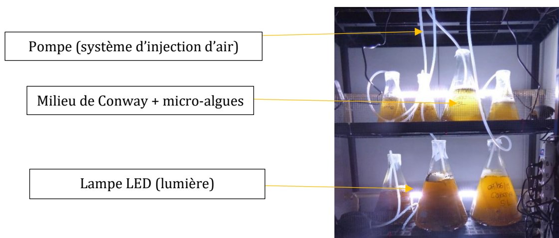
Figure 27. Dispositif expérimental de la culture de la diatomée « C. closterium »
