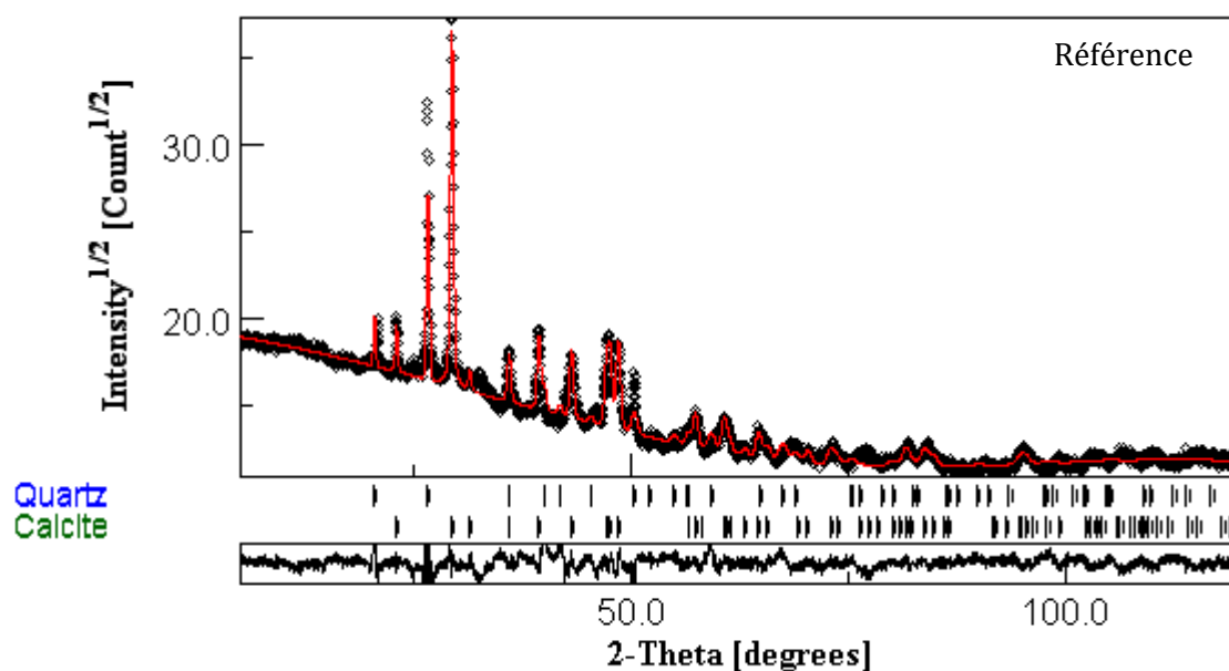
Figure 70. Spectre DRX de la surface d'un mortier référence (avant immersion)
