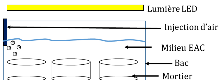
Figure 49. Dispositif expérimental installé en laboratoire pour le milieu EAC
