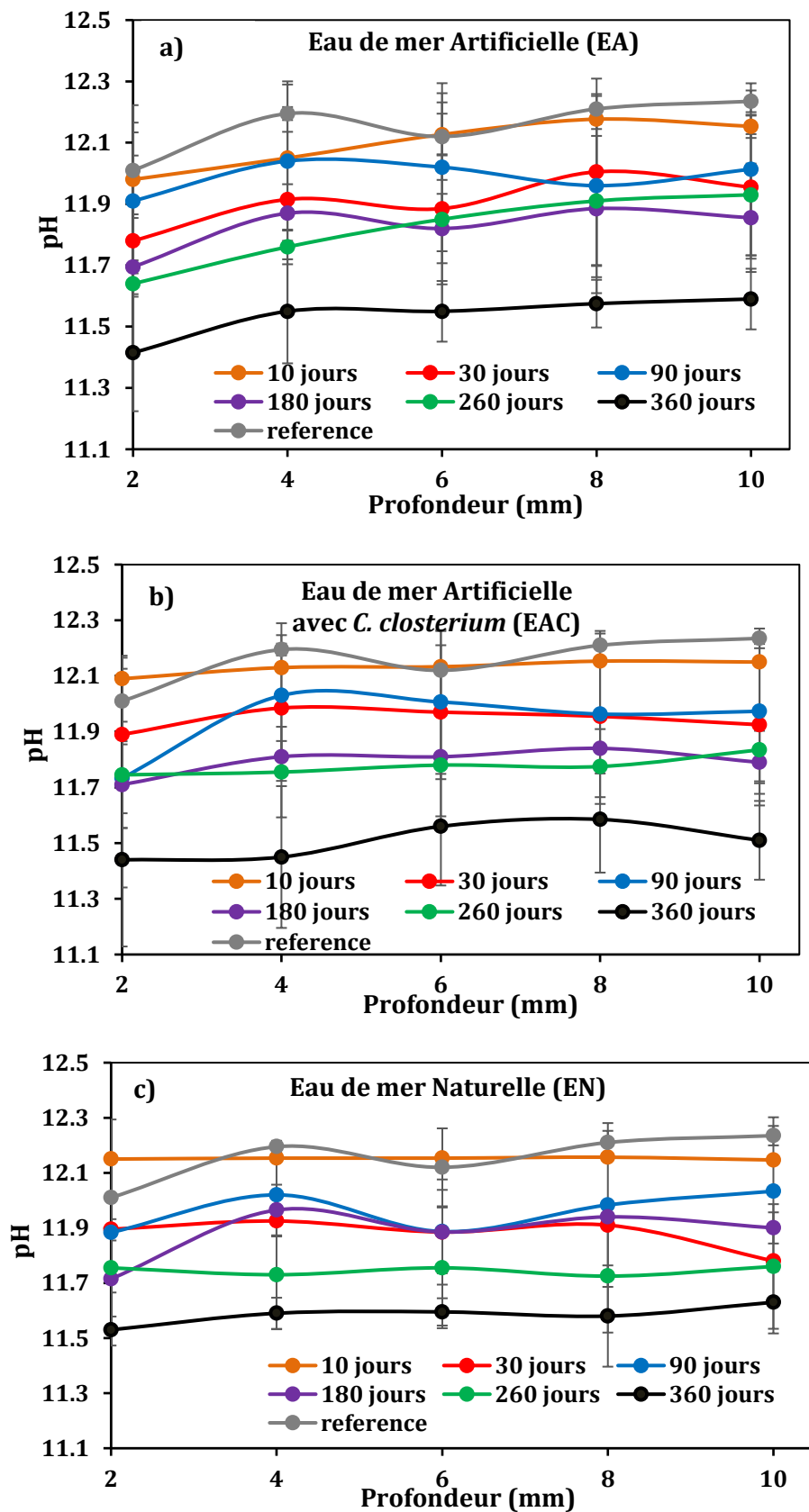
Figure 60. Evolution du pH du mortier en fonction de la durée d'immersion et de la profondeur dans différents milieux en : (a) eau de mer artificielle ; (b) eau de mer artificielle + C. closterium ; (c) eau de mer naturelle
