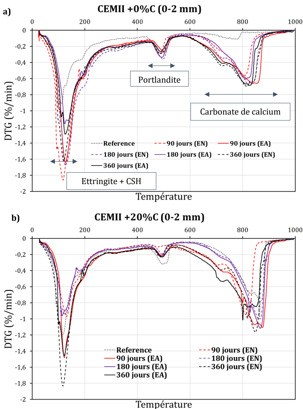
Figure 86. Courbes DTG (%/min) de bétons CEMII +0%C et CEMII +20%C référence et immergés dans les 2 environnements étudiés (EN et EA) à 90 -180 et 360 jours à une profondeur de 0 – 2 mm
