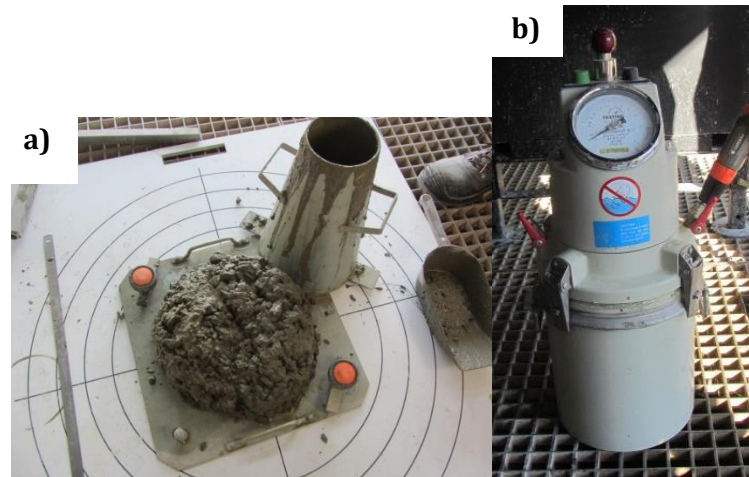
Figure 17. Mesure au cône d'Abrams (a) ; Mesure de l'air occlus (b)
