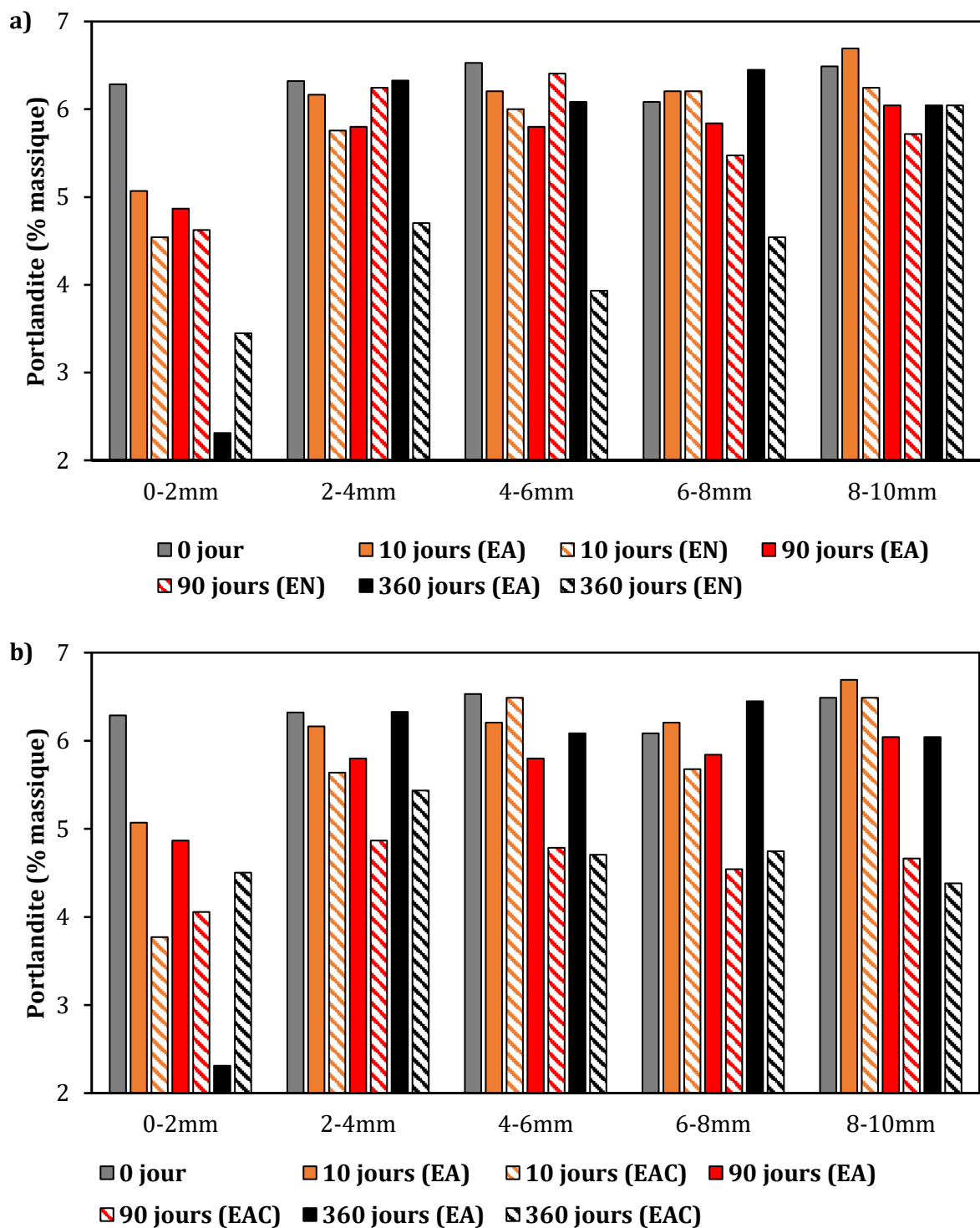
Figure 63. Evolution de la portlandite (% massique) dans les mortiers immergés en Eau de mer Naturelle + Biofilm naturel (EN) (a) et en Eau de mer Artificielle avec C. closterium (EAC) (b) comparé au mortier référence et immergé en Eau de mer Artificielle (EA) à différentes profondeurs après 10, 90 et 360 jours d'immersion
