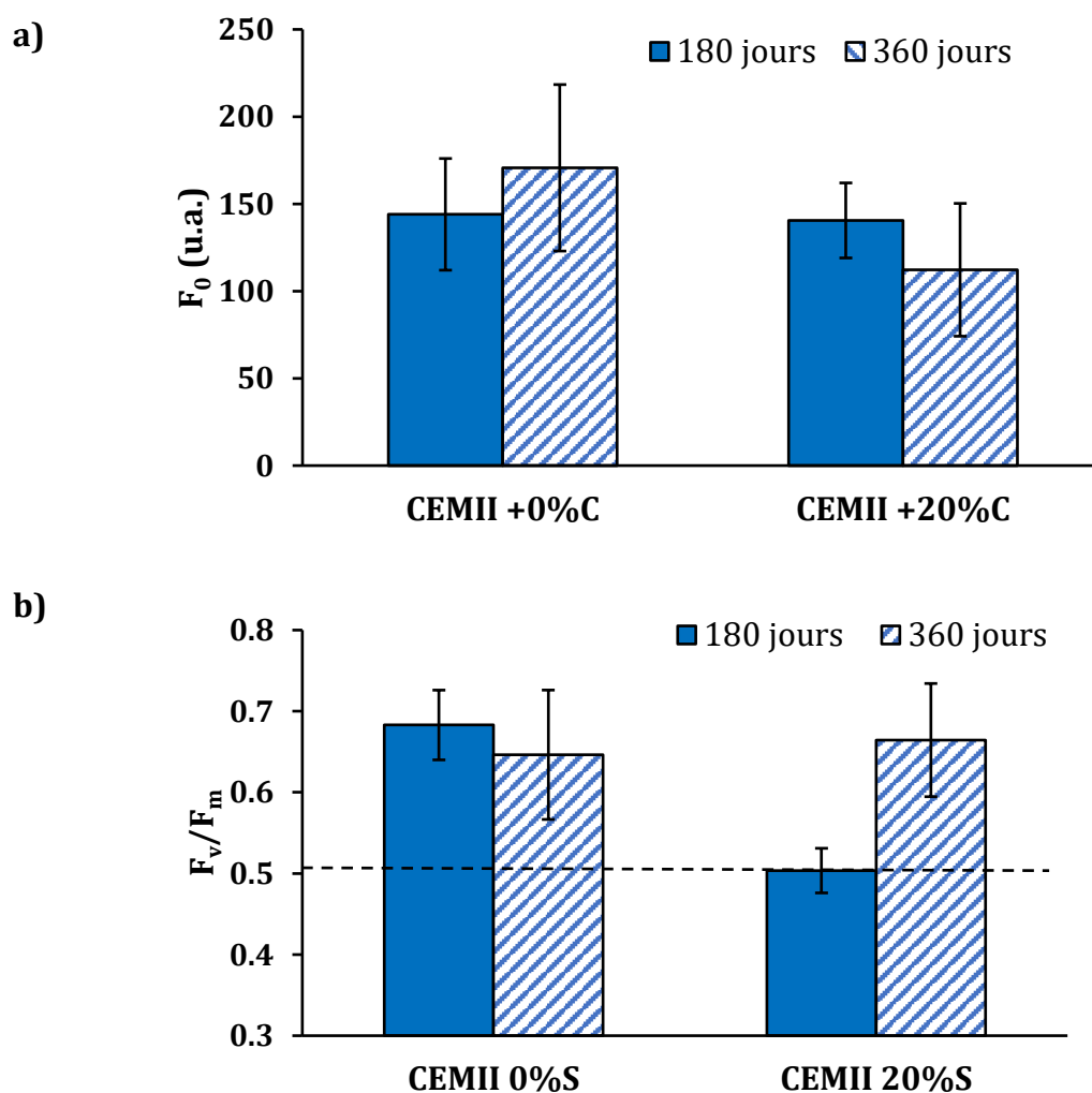
Figure 83. Dynamique de la colonisation par le biofilm microphytobenthique en fonction du type de béton. (a) Biomasse chlorophyllienne F_0 du microphytobenthos ; (b) Indice F_v/F_m Rendement quantique maximum du PSII (ie. Indice d'état physiologique)
