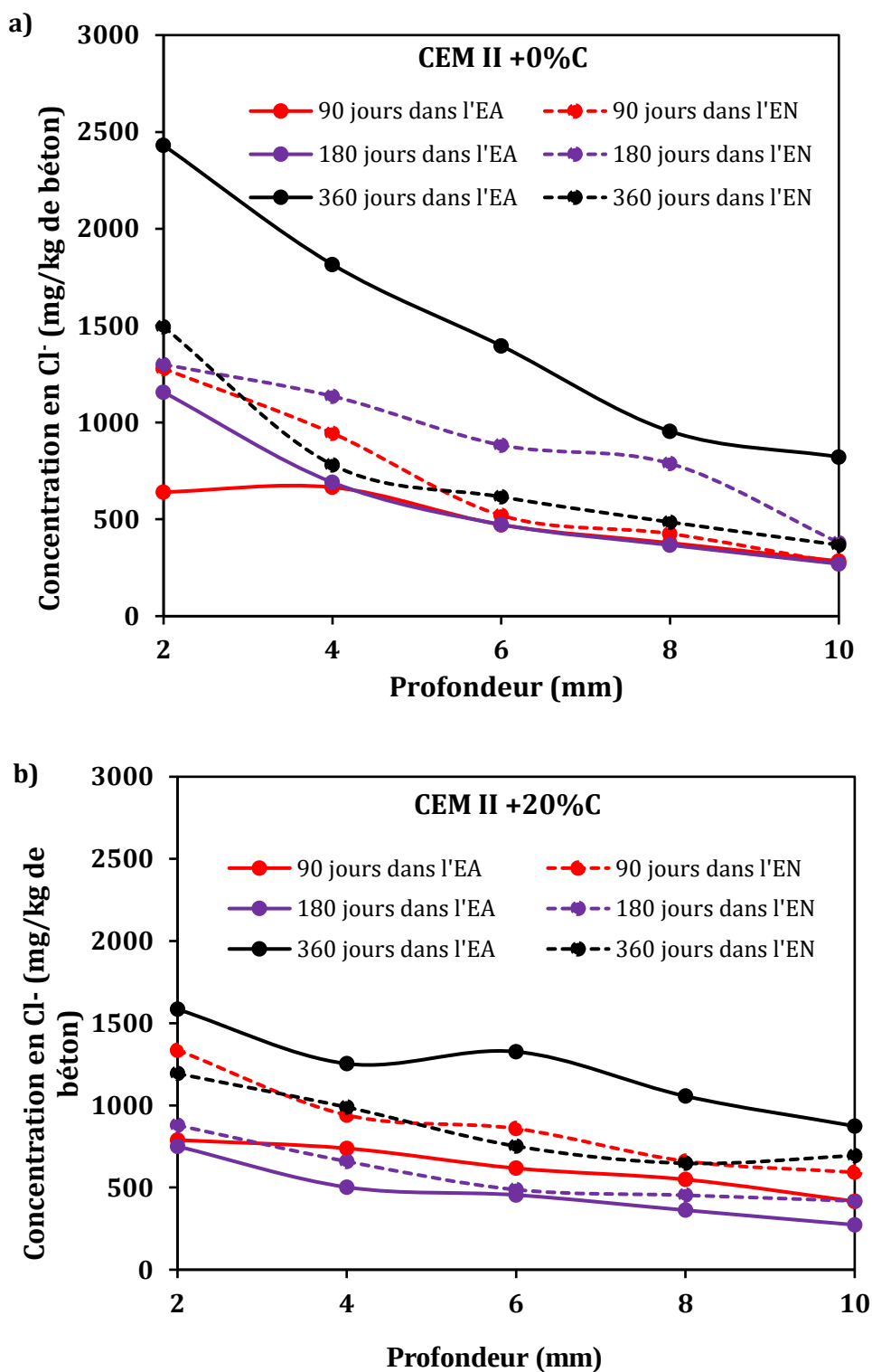
Figure 87. Profils de pénétration des ions chlorure libres des échantillons jusqu'à 10 mm de profondeur, par rapport aux temps d'immersion dans de l'eau de mer artificielle (EA) (ligne pleine) dans de l'eau de mer naturelle (EN) (ligne pointillée) pour le béton CEM II +0%C (a) et le béton CEMII +20%C (b)
