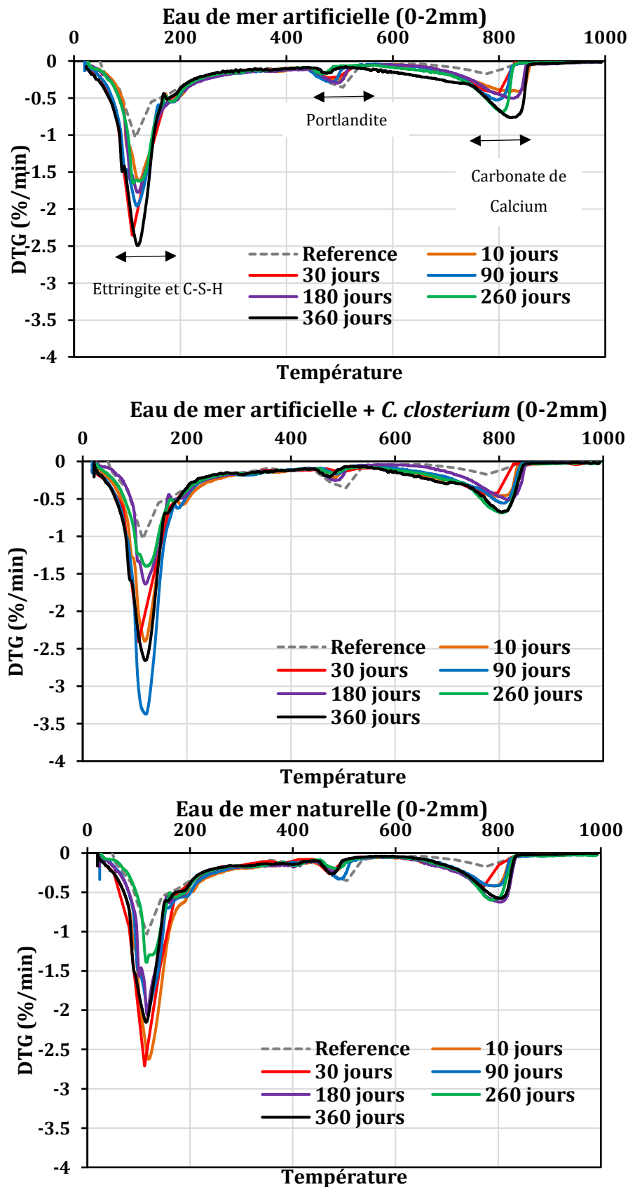
Figure 62. Courbes DTG (%/min) des mortiers référence et immergées, dans les trois milieux étudiés après 10 -30-90-180-260-360 jours d'immersion (profondeur étudiée : 0-2 mm)
