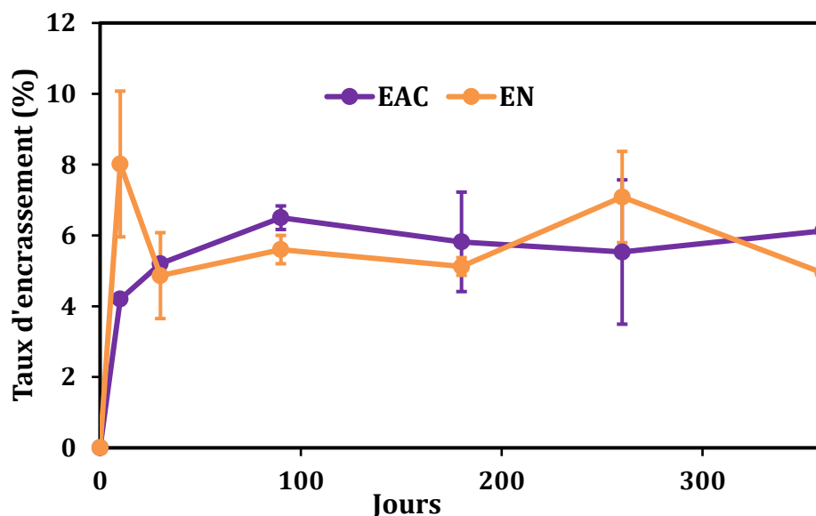
Figure 53. Taux d'encrassement (%) du mortier au cours du temps dans l'environnement EAC et EN
