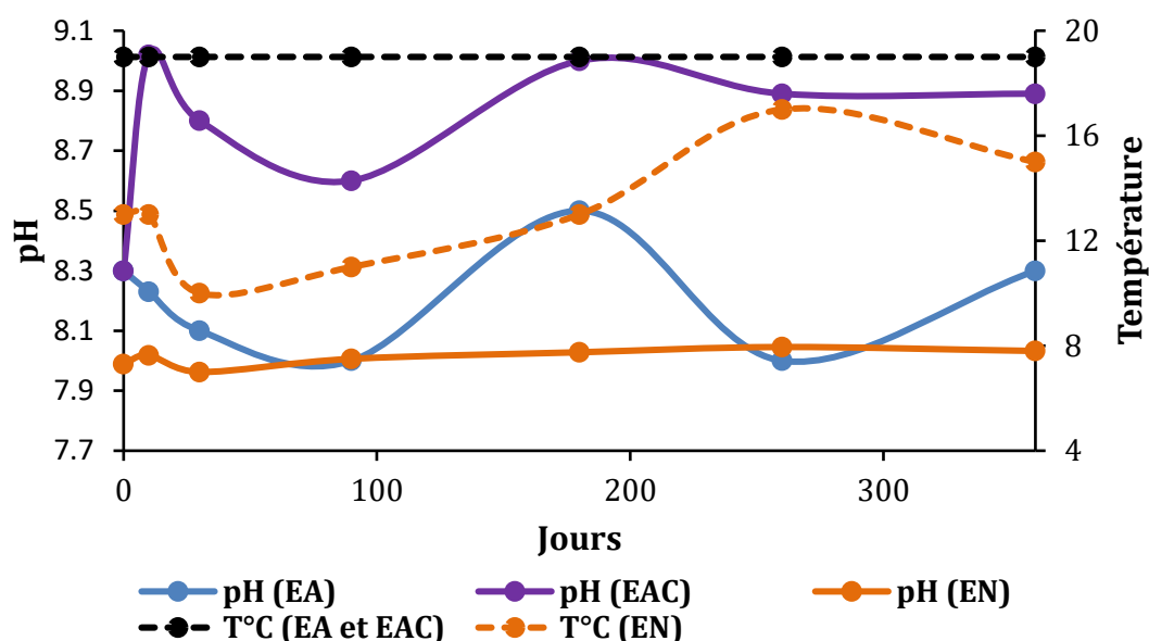
Figure 51. Evolution du pH (ligne en gras) et de la température (ligne en pointillé) en fonction de la durée et du milieu d'immersion (EA, EAC et EN)
