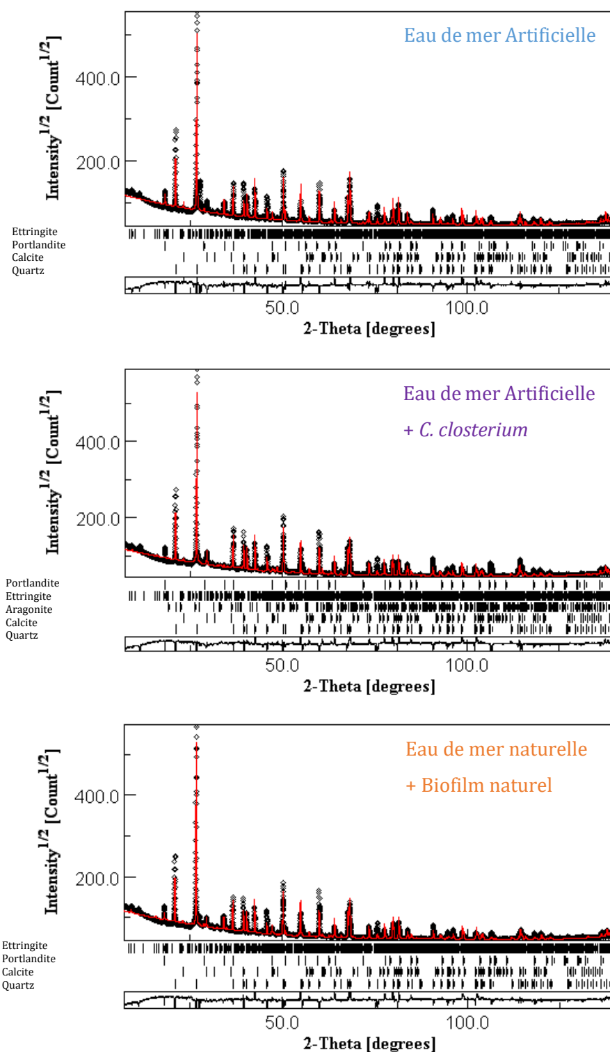
Figure 74. Spectres DRX de poudre de mortier immergé après 90 jours d'immersion dans les trois conditions étudiées (EA, EAC et EN)
