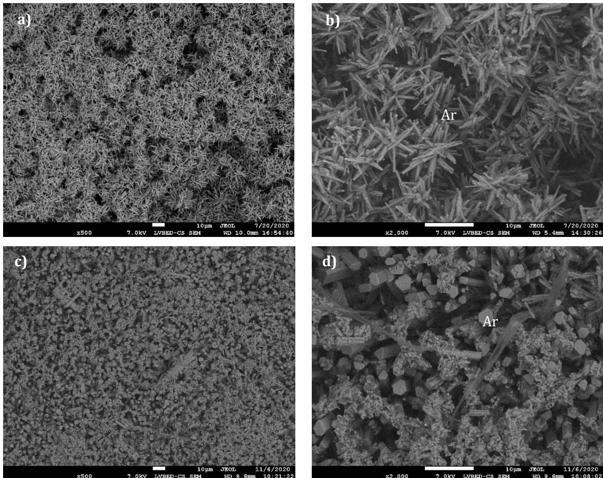
Figure 66. Observations MEB du mortier immergé en Eau de mer Artificielle après 90 (a-b) et 360 jours (c-d) d'immersion (Ar : Aragonite)
