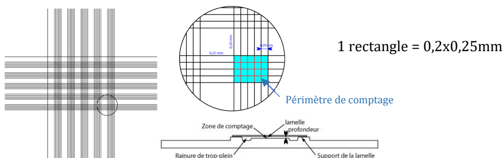
Figure 37. Cellule de Malassez
