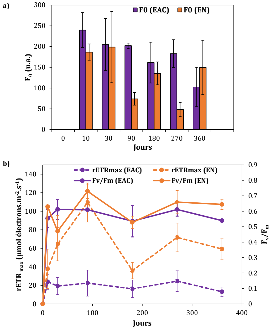
Figure 52. Dynamique de la colonisation par le biofilm microphytobenthique sur du mortier en fonction du temps dans les deux milieux étudiés (en Eau de mer Artificielle + biofilm de C. closterium + nutriments (EAC) (ligne en gras) et en Eau de mer naturelle + biofilm naturel (EN) (ligne en pointillée)) : (a) Biomasse chlorophyllienne F_0 du microphytobenthos et indice F_v/F_m Rendement quantique maximum du PSII (ie. Indice d'état physiologique) ; (b) Capacité photosynthétique maximale du biofilm ( rETR_{max} , \mu\text{mol. e}^{-}\cdot\text{m}^{-2}\cdot\text{s}^{-1} )
