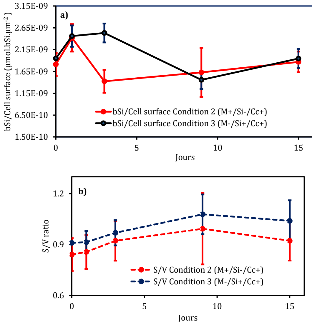
Figure 44. Taux de production de la silice par les diatomées i.e. degré de silicification (bSi par surface cellulaire) (a) et rapport S/V dans la condition 2 (M+/Si-/Cc+) et 3 (M-/Si+/Cc+) (b)
