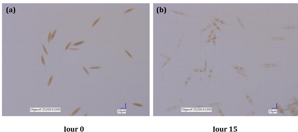
Figure 43. Observation microscopique (S200×1000) des chloroplastes de C. closterium dans la solution initiale au jour 0 (a) et au jour 15 (b) dans la condition 2 (M+/Si-/Cc+).
