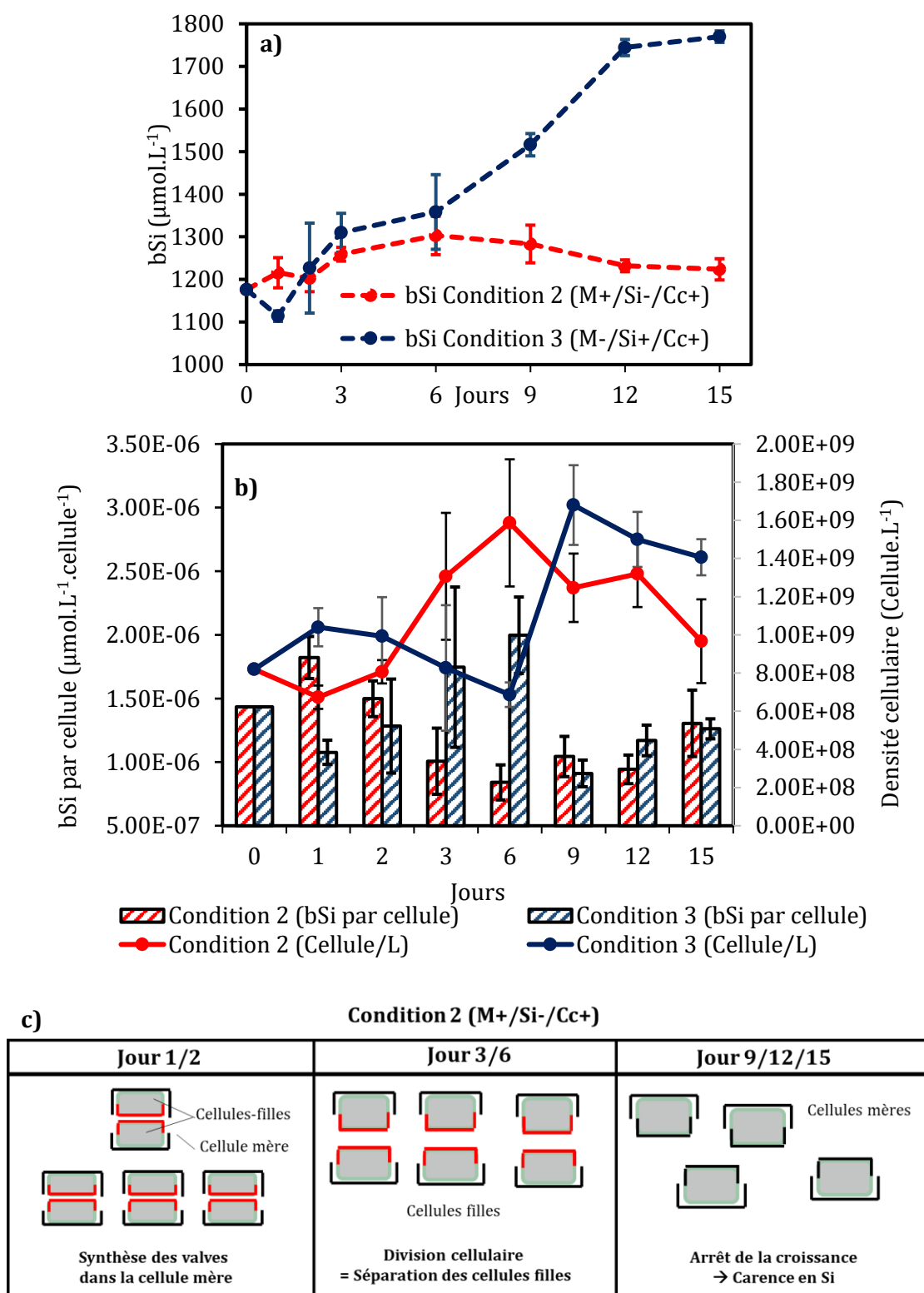
Figure 41. Concentration de silice biogène (bSi), i.e. le taux de formation des frustules ( \mu\text{mol.L}^{-1} ), et densité cellulaire ( \text{cellule.L}^{-1} ) de C. closterium en fonction du temps (a) ; teneur en bSi par cellule ( \mu\text{mol.L}^{-1}.\text{cellule}^{-1} ) (b) ; Schéma simplifié du cycle cellulaire des diatomées cultivées dans la condition 2 au cours du temps (c).
