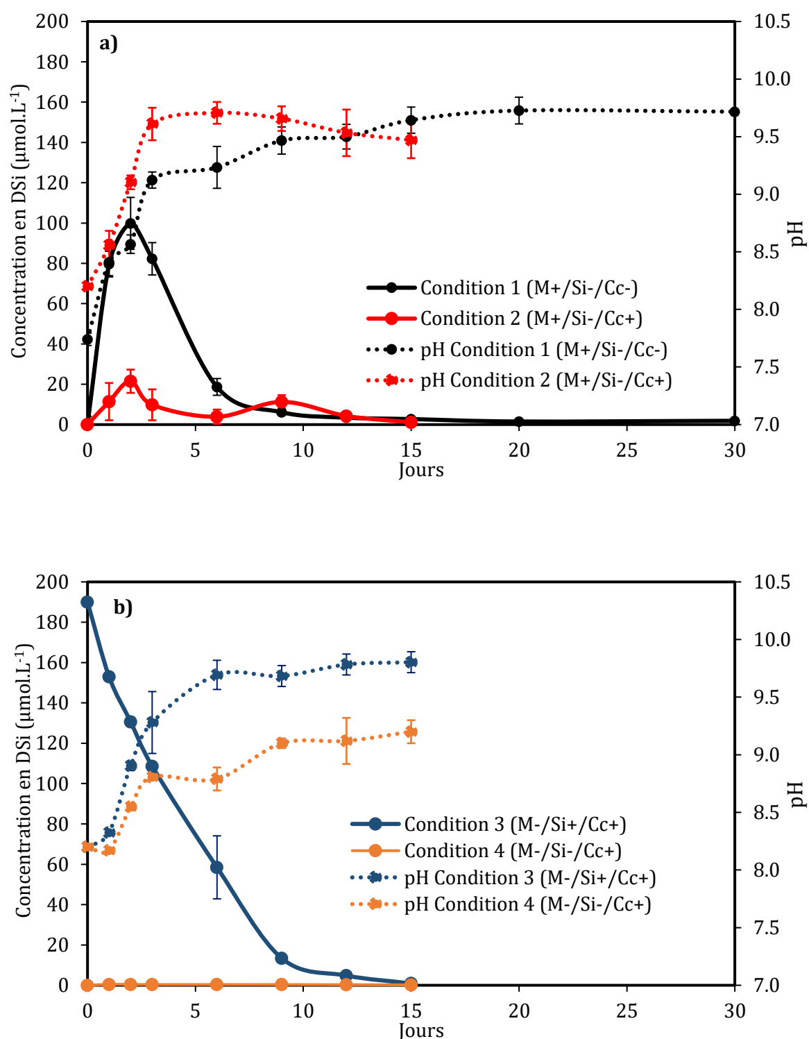
Figure 39. Concentration en silice dissoute et pH mesurés dans la condition 1 (M+/Si-/Cc-) et condition 2 (M+/Si-/Cc+) (a) dans les conditions de contrôle (condition 3 (M-/Si+/Cc+) et condition 4 (M-/Si-/Cc+)) (b) . Les moyennes \pm la plage de trois répétitions sont indiquées.
