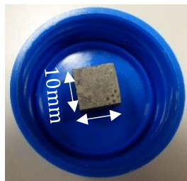
Figure 34. Taille des échantillons de mortier étudiés (10 mm × 10 mm × 5 mm).
